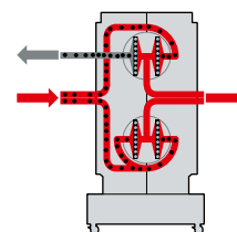
Обратная промывка во время производственного процесса
